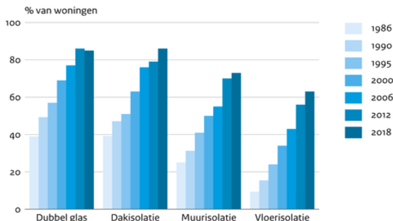
Figuur 4 - Isolatiegraad van de Nederlandse woningvoorraad door de jaren heen
