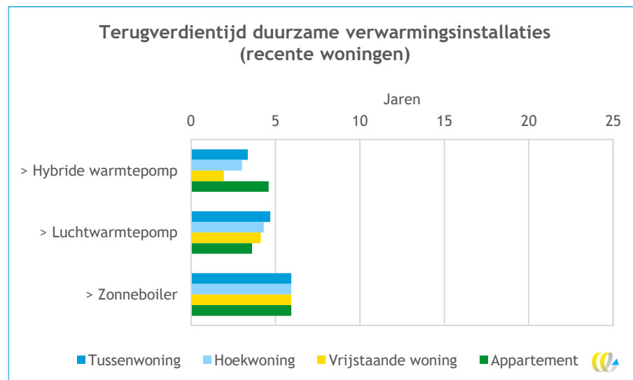
Figuur 12 - Terugverdiertijden duurzame verwarmingsinstallaties bij huidige energieprijsen
