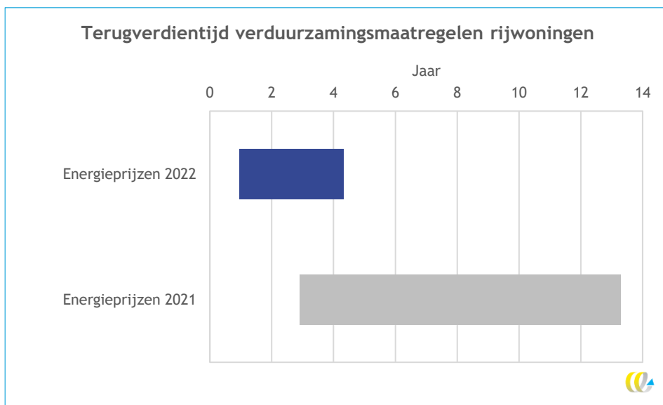
Figuur 6 - Invloed van prijsniveau op de terugverdiertijden van isolatiemaatregelen voor een vooroorlogse rijwoning.
